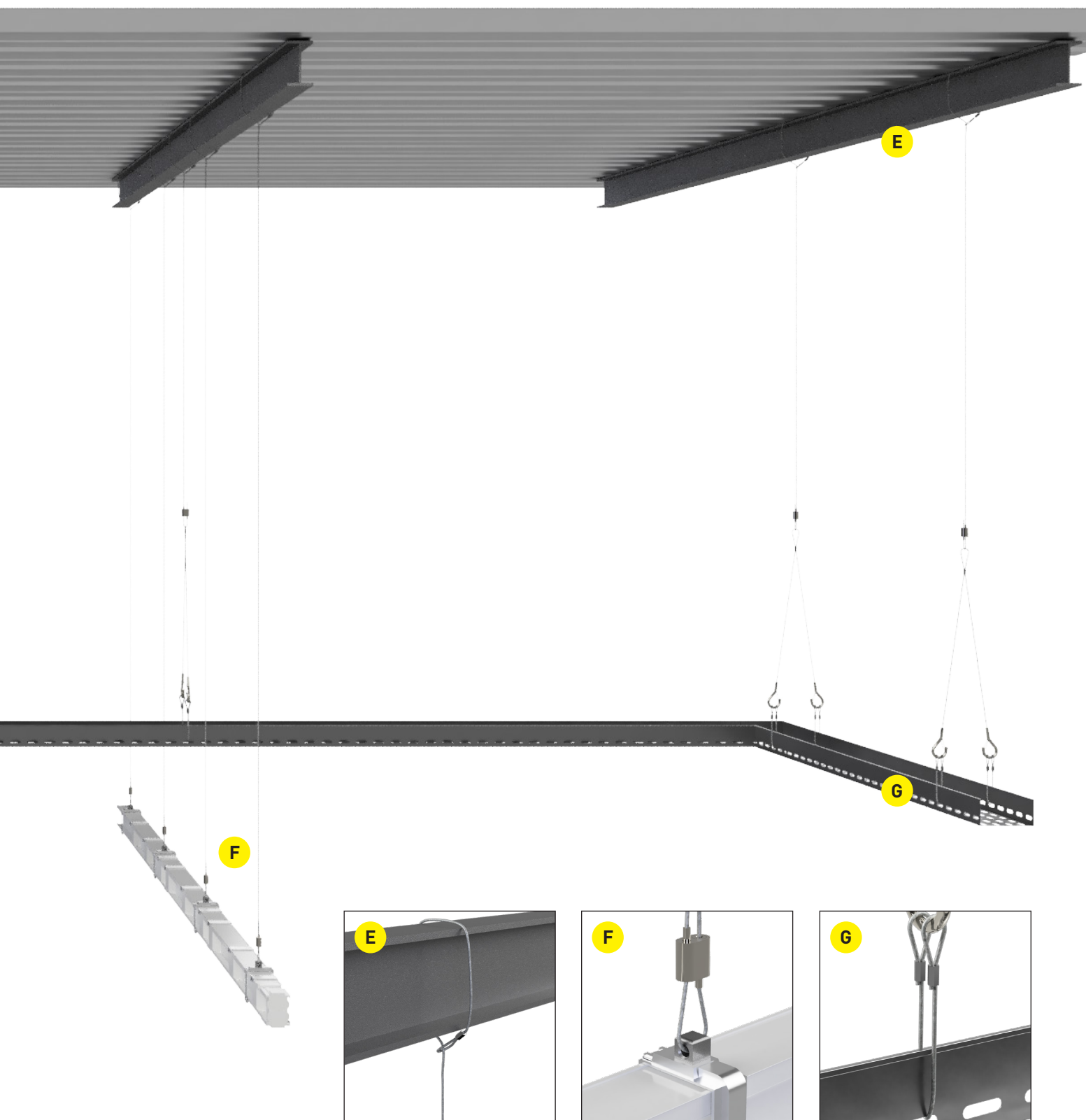
KIT DBFM - Terminaison boucle Page 28
