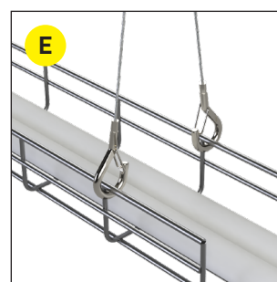
Accroche V Page 34
