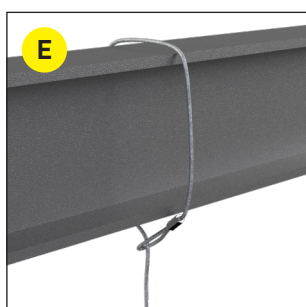
KIT DBFM - Terminaison boucle Page 28
