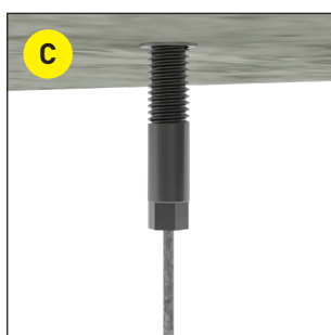
KIT DBFM -Terminaison filetée Page 28
